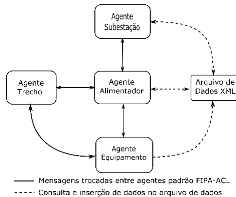
Figura 1. Diagrama de blocos representando comunicação entre agentes e com acesso ao arquivo de dados XML.
